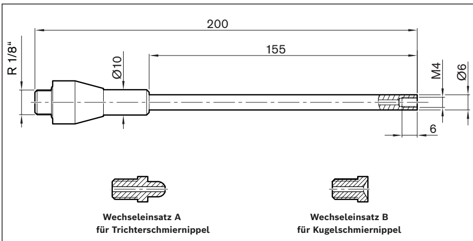
Düsenrohr
