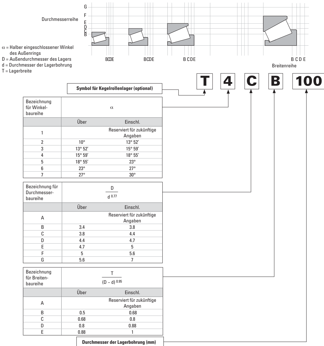
Abb. 32: ISO 355-Teilenummernsystem.
