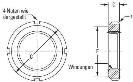
Abb. 49: Kontermütern (Windungen gemäß ISO 965/1, Klasse 5H).
