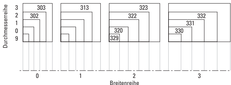
Abb. 31: Original ISO-Teilenummernsystem.
