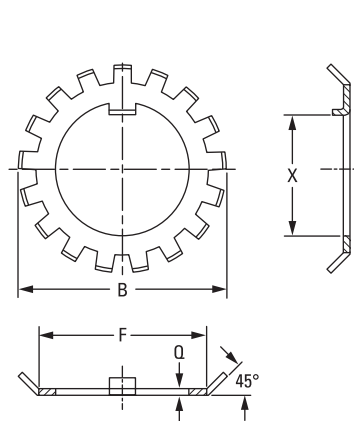
Abb. 53: Sicherungsringe.
