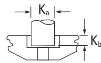
Verschlussbolzen für CD-Außenlaufbahn.
