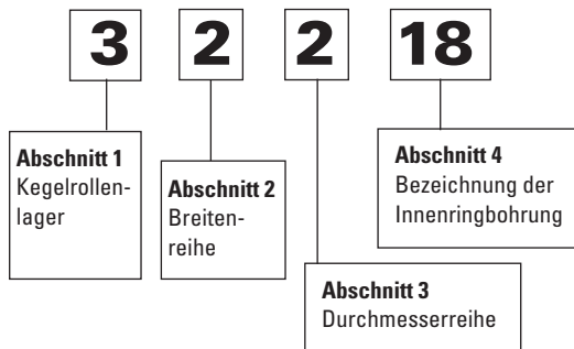
Abb. 30: Nomenklatur des Teilenummernsystems für originale ISO-Abmessungen.
