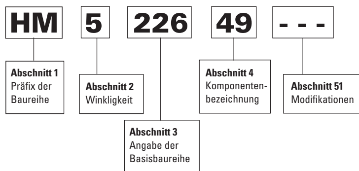
Abb. 26: Nomenklatur des ABMA-Teilenummernsystems für Zollabmessungen.
