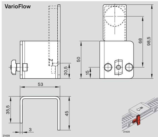
Montagesatz ID 200/MS-5
