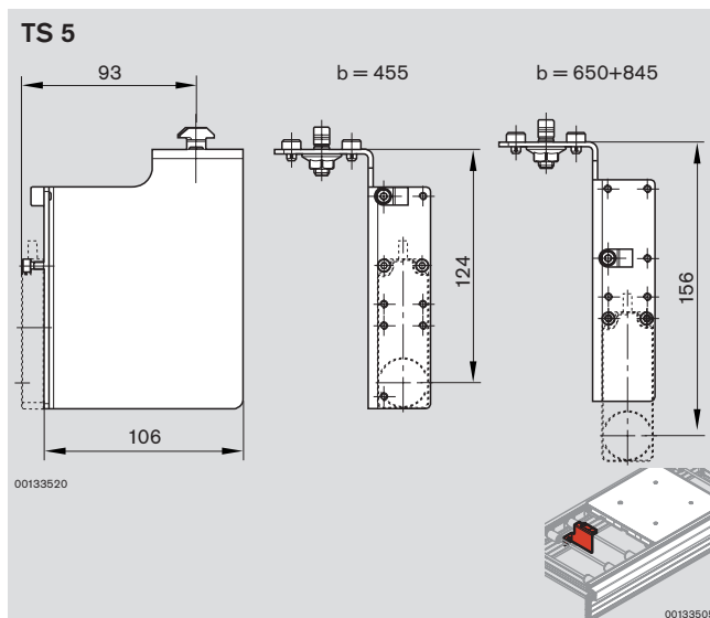
Montagesatz ID 200/MS-7
