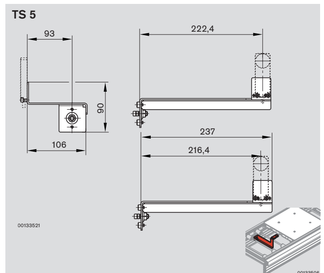
Montagesatz ID 200/MS-8
